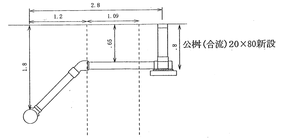
断面図 S=1/50
