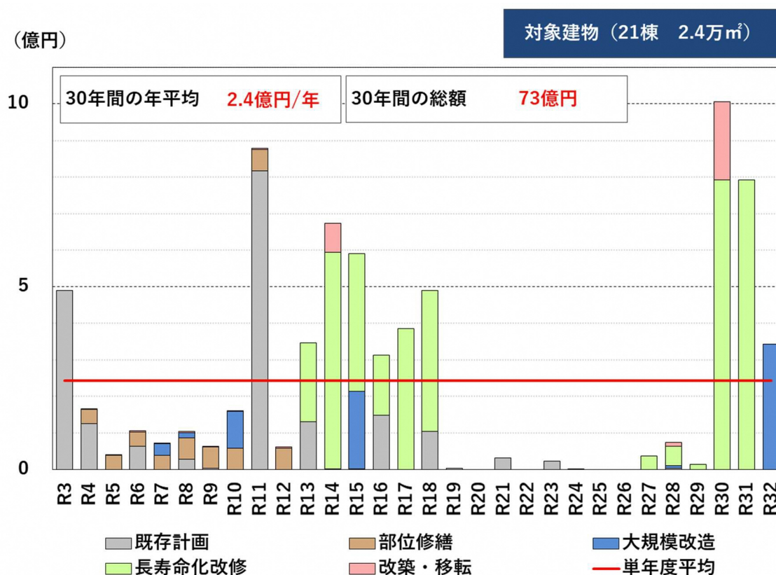
図 15 維持・更新費用の見込み（長寿命化）
