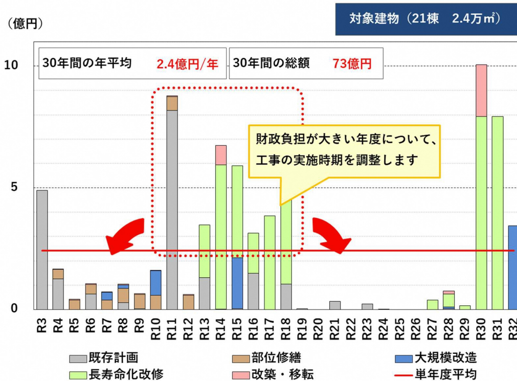
図 16 平準化のイメージ
