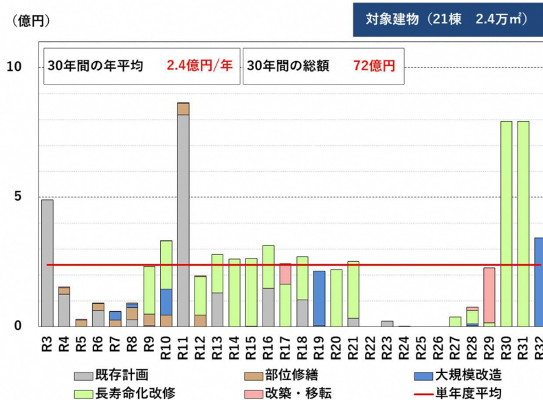
図 18 平準化の結果
