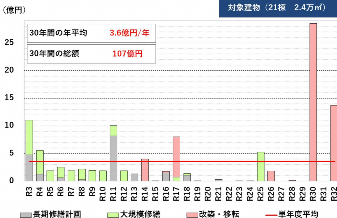
図 13 維持・更新費用の見込み (総合管理計画)
